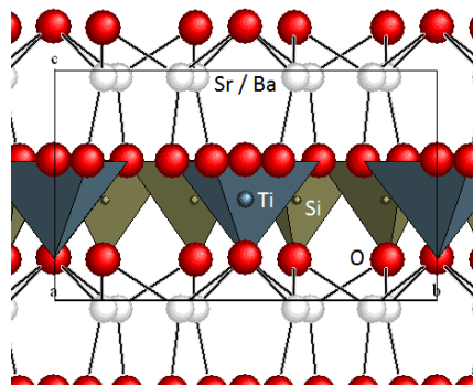
Fig. 1. Fresnoite structure
